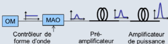
Architecture MOPFA (master oscillator - power fiber amplifier). OM : oscillateur maître, MAO : modulateur acousto-optique.
