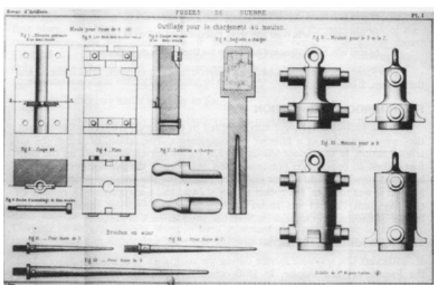
Mouton (réf. Fusées de guerre - Pralon - 1883)
