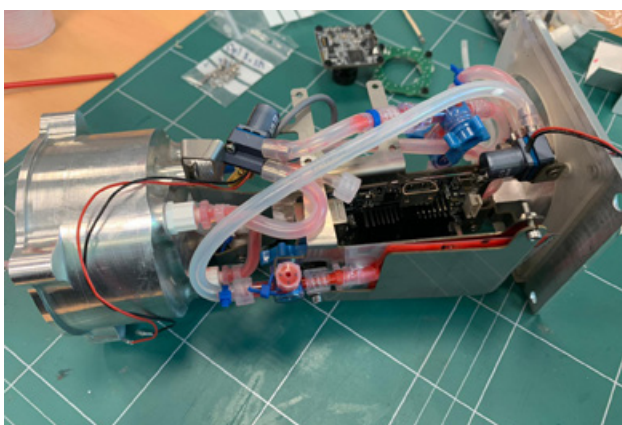
Figure 4 : Cube assemblé sans boîte
