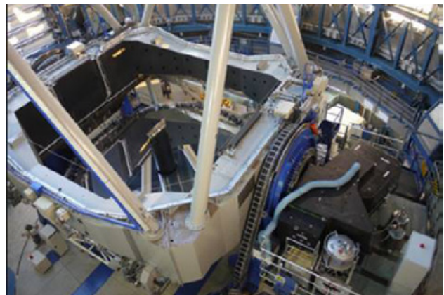
Figure 1 : L'instrument SPHERE installé au foyer Nasmyth du VLT
