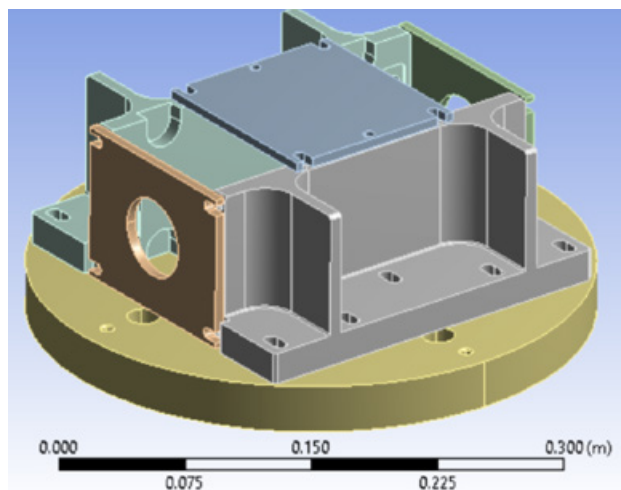
Figure 5 : Adaptateur et un disque de plaque
