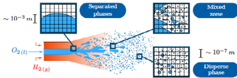
Figure 2 : Organisations d'écoulement et échelles de l'atomisation de jet par injection cryogénique en conditions sous-critiques.
