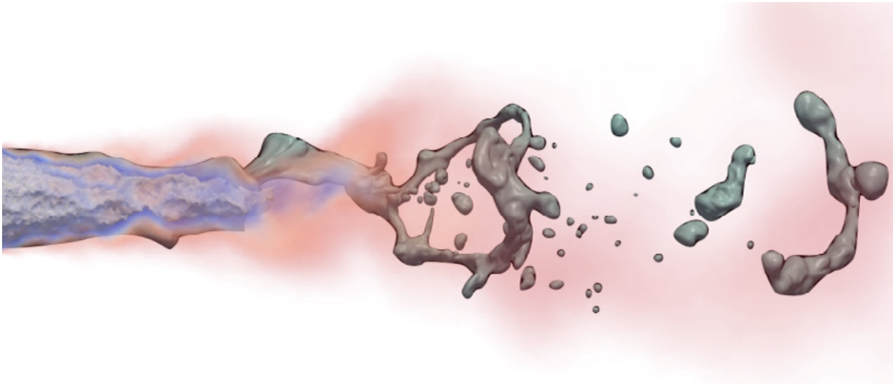
Figure 3 : Dard liquide obtenu avec le modèle d'ordre réduit implémenté dans CEDRE (couleur) comparé aux résultats du code DNS ARCHER (gris).
