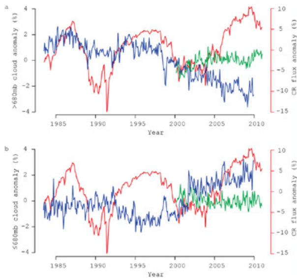
Figure 5 : Corrélation entre la couverture nuageuse à basse (a) et moyenne (b) altitude et les rayons cosmiques dans l'intervalle de temps 1985–2010 [31].
