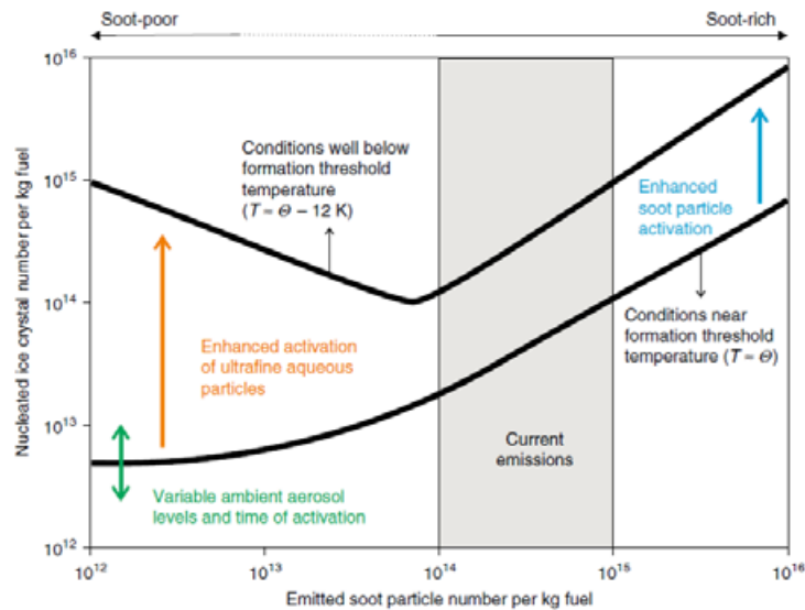
Figure 9 : Nombre de cristaux de glace formés par kg de carburant en fonction du nombre de particules de suies émises par kg de carburant pour deux températures ambiantes. (Extrait de Kärcher, 2018).
