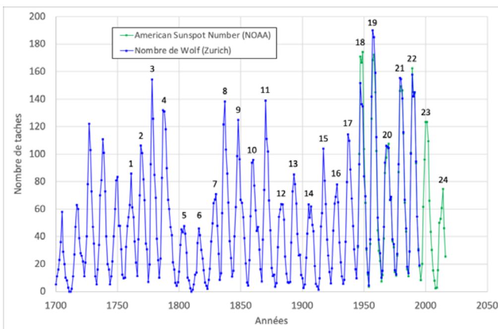
Figure 2 : Variation de l'activité solaire estimée par le nombre de Wolf R_z (données [4] et NOAA).
