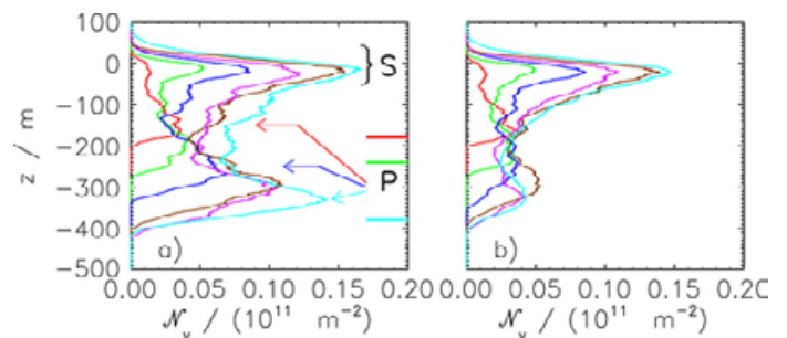
Figure 7 : Profils verticaux du nombre de cristaux de glace intégré le long du contrail 4 minutes après l'émission pour deux saturations par rapport à la glace (140 % à gauche et 120 % à droite). La position des tourbillons primaire et secondaire est notée P et S respectivement, sur le graphique de gauche. La fréquence de Brunt-Vaisala est de 1,15 \cdot 10^{-2} \text{s}^{-1} . L'altitude de croisière est z = 0 . (Unterstrasser et Görsch, 2014).
