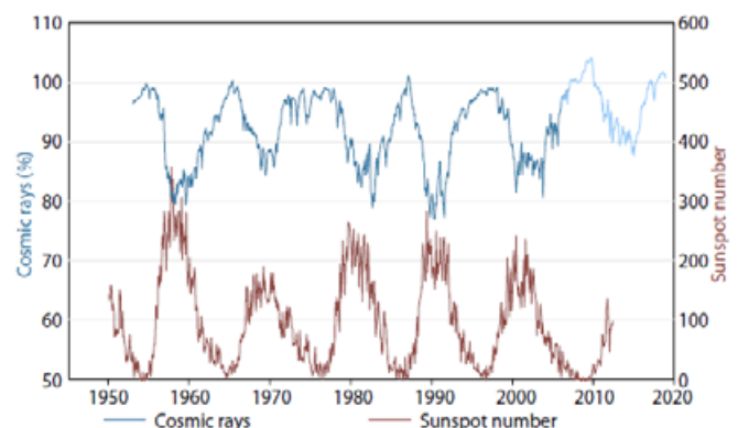
Figure 4 : Anti-corrélation du rayonnement cosmique avec l'activité solaire mesurée par le nombre de taches ([40]).
