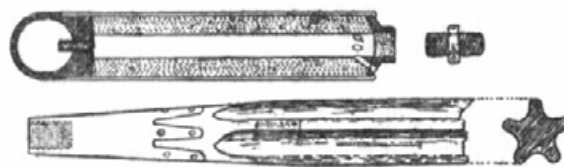
Fusée de 5 (1849) [note 8]
