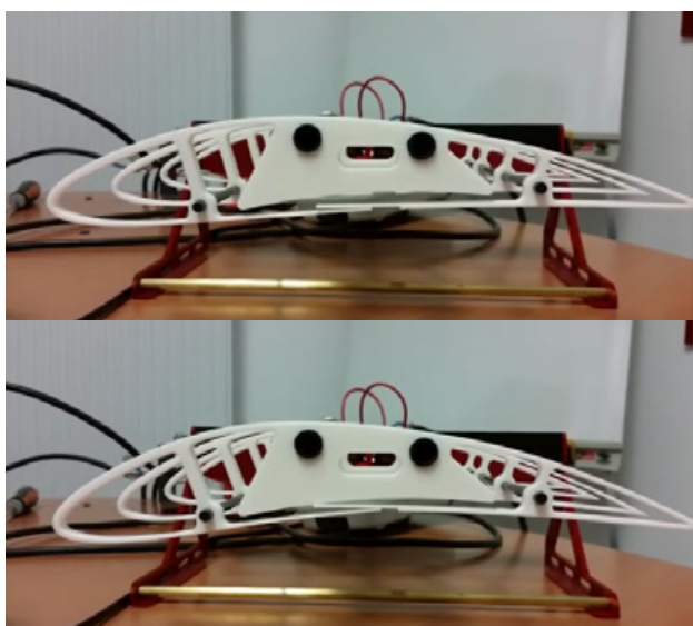
Figure 4 : Wing morphing activé par un AMF @Nimesis
