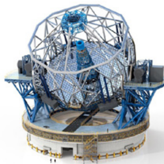
Figure 5.1 : L'ELT : un Dôme de 74 m de haut, une base de 89m de diamètre, 5000 tonnes, un miroir primaire de 39m de diamètre composé de 798 segments hexagonaux de 1.4m positionnés avec une précision sub-micrométrique.
