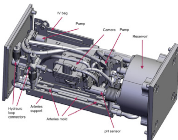
Figure 3 : Modèle 3D de la structure interne du Cube
