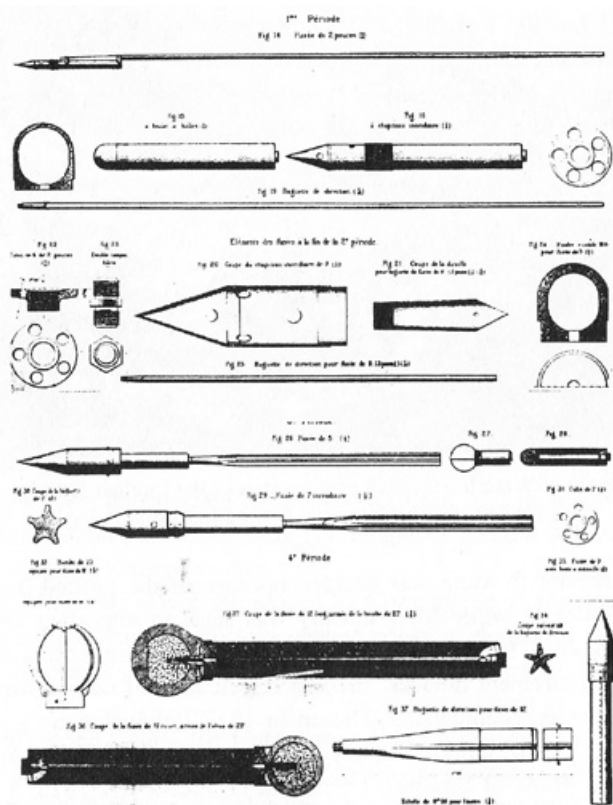
Évolution des fusées françaises, de Toulouse (1818) à Metz (1833, 1849/50, 1854/56) [Cne Pralon- Revue d'Artillerie 1882]
