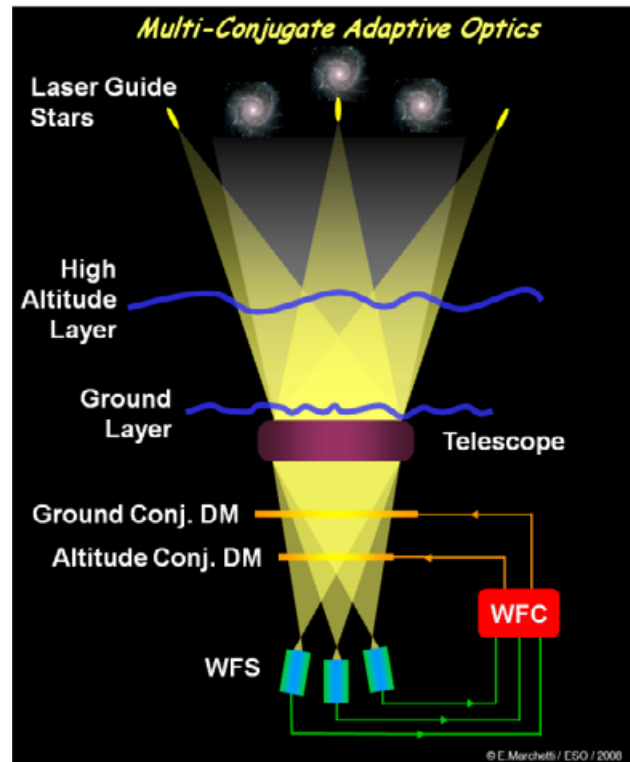
Figure 4 : Le concept d'OA tomographique assistée par laser. Plusieurs étoiles artificielles créées en excitant des atomes de sodium à 90 km d'altitude servent de référence pour une mesure bidimensionnelle du front d'onde dans plusieurs directions permettant une reconstruction tridimensionnelle du volume turbulent. Ce dernier étant ensuite corrigé grâce à plusieurs miroirs conjugués optiquement à différentes altitudes
