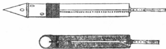
Fusées de 3 pouces 6 lignes construites par Bedford à Metz en 1827 [note 10]
