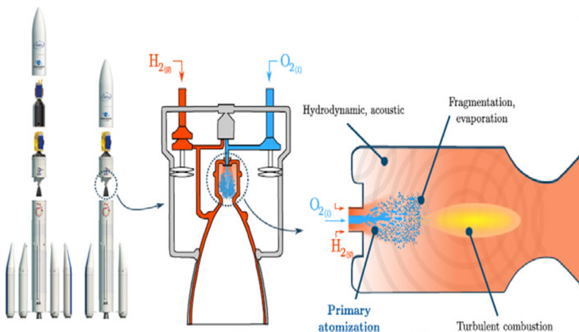
Figure 1 : Représentation de l'atomisation de l'oxygène liquide O_{2(l)} dans l'hydrogène gazeux H_{2(g)} au sein de la chambre de combustion des moteurs cryogéniques équipant Ariane 6.
