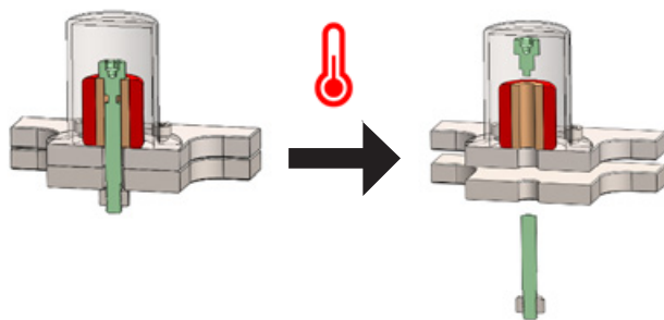
Figure 5 : Schéma de principe d'un Triggy @Nimesis
