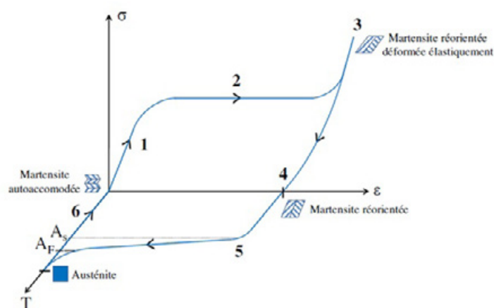
Figure 1 : Représentation schématique de l'effet mémoire de forme
