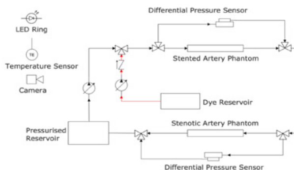
Figure 1 : Schéma de circuit hydraulique
