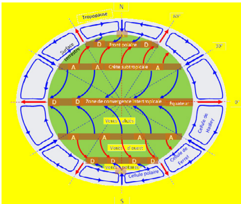
Figure 9 : Structure schématique de l'atmosphère terrestre due à la circulation générale. Les cellules convectives sont représentées en coupe sur la troposphère bleue. Les directions des vents dans la basse troposphère sont indiquées en rouge et en bleu en projection sur le disque terrestre vert. La rotation cause un aplatissement du globe terrestre et de la troposphère, celle-ci étant plus mince aux pôles (8 km environ) qu'à l'équateur (16 km environ). Par souci de clarté, l'épaisseur de la troposphère (entre la surface terrestre et la tropopause) est exagérée par rapport au rayon terrestre (A : anticyclone ; D : dépression).
