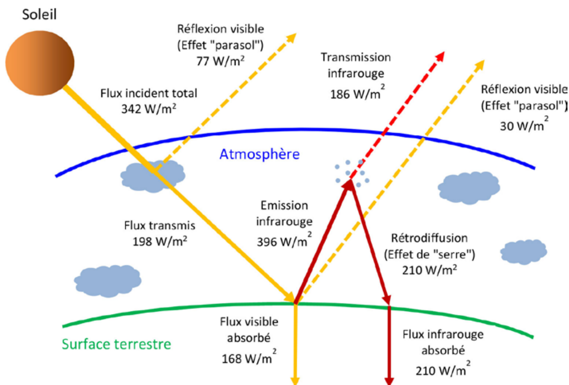
Figure 10 : Représentation schématique du bilan énergétique dans l'atmosphère terrestre (Tableau 1). Les directions des rayons sont indicatives.
