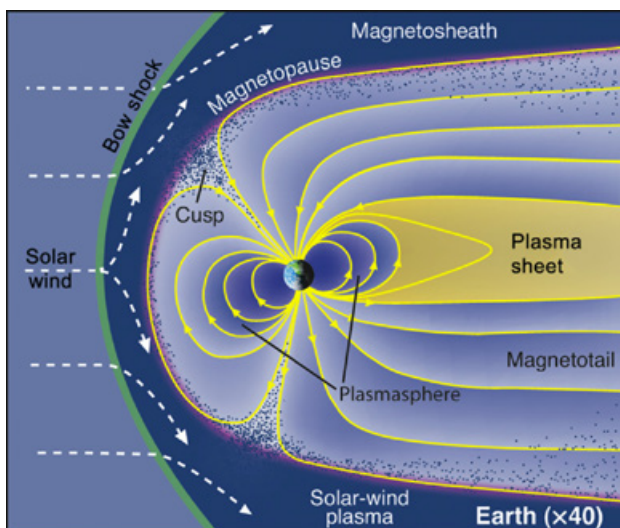
Figure 8 : Champ magnétique terrestre montrant le vent solaire, l'arc de choc et la magnétosphère limitée par la magnétopause (19). La Terre n'est pas à l'échelle ( \times 40 ).
