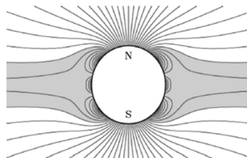
Figure 1 : Champ magnétique solaire. Coupe dans un plan méridien ([9]).
