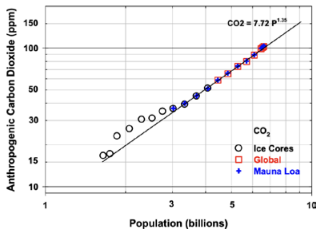
Figure 12 – Corrélation entre la concentration en CO 2 supposée d'origine humaine et la population mondiale (billion = milliard) [27].
