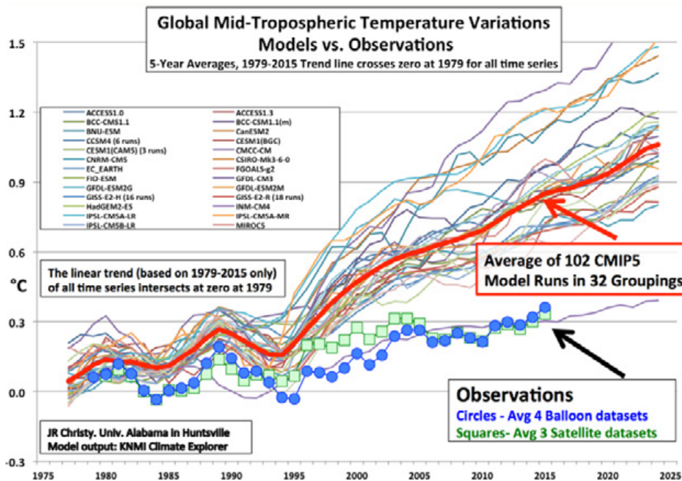
Figure 11 : Comparaison entre les simulations numériques du GIEC et les observations par satellite et ballon [18].
