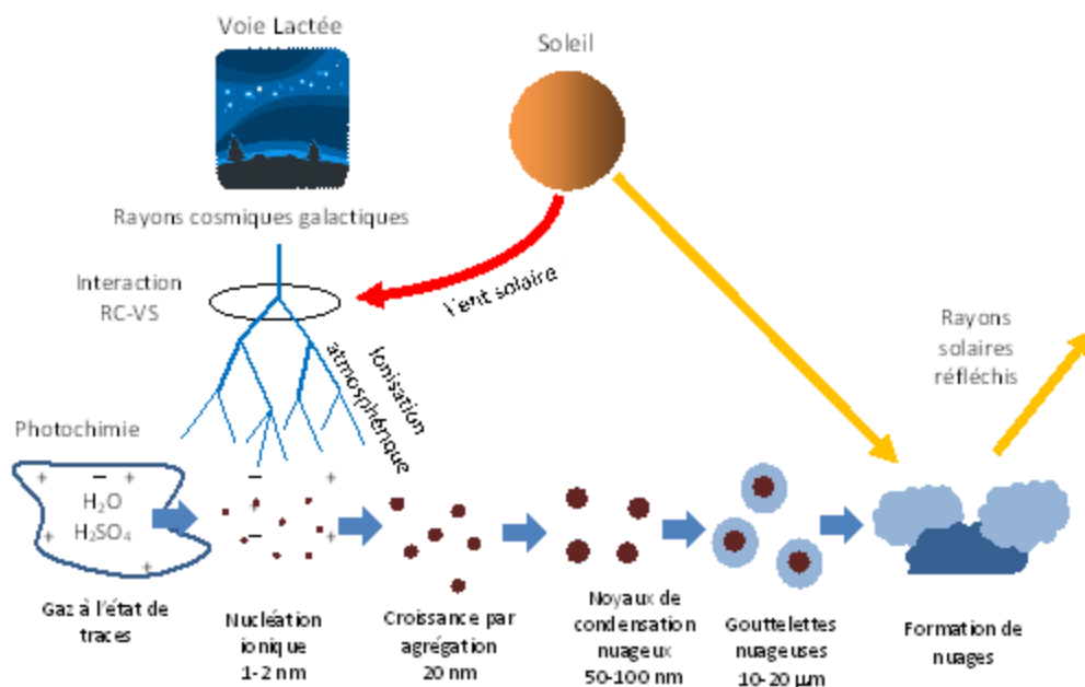
Figure 6 : Mécanisme de nucléation activé par les rayons cosmiques (d'après [40]).
