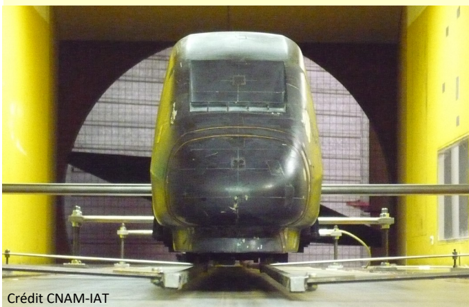
Soufflerie Veine Longue (SVL), 1972.
