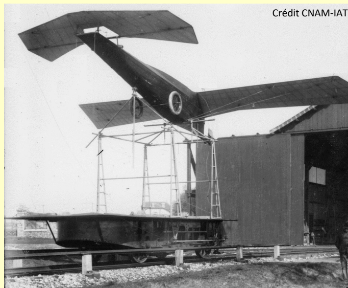
Chariot d'essais avec modèle d'avion.
